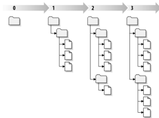
Pav. 1 Subversijos medžio istorija (paimta iš http://svnbook.red-bean.com/en/1.4/images/ch02dia7.png , pagal CC licenziją)
